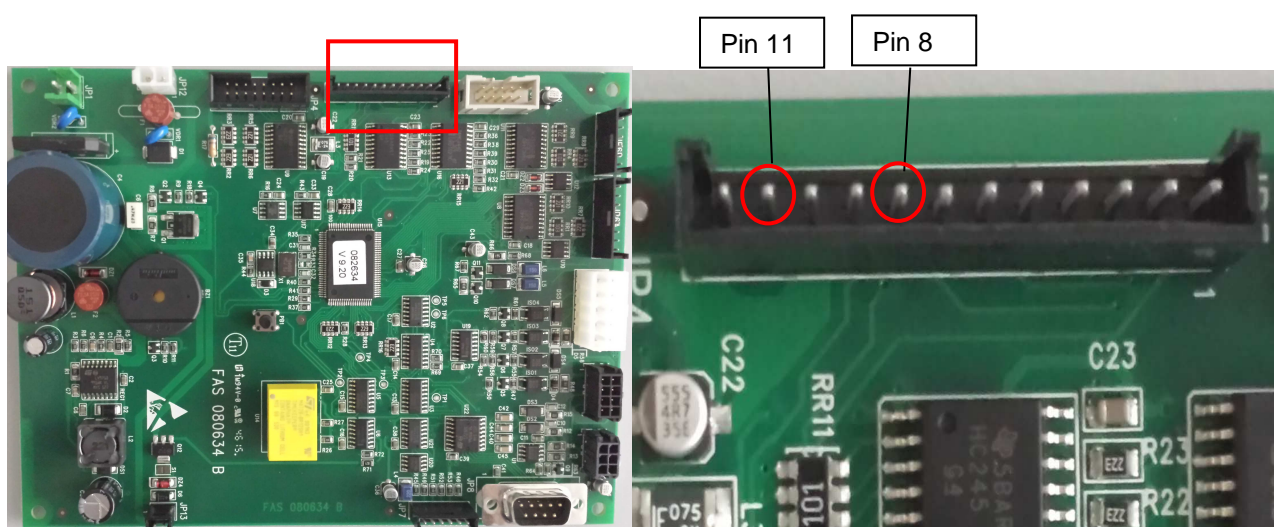
Hauptplatine
